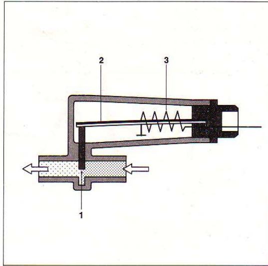
29. ábra. Pótlevegőrekesz 1 Légcsatorna a to- lórészessel 2 Bimetall 3 Villamos fűtés
