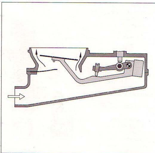
13. ábra. Emelőáramú légmennyiségmérő működési helyzetben, egyszerűsítve
