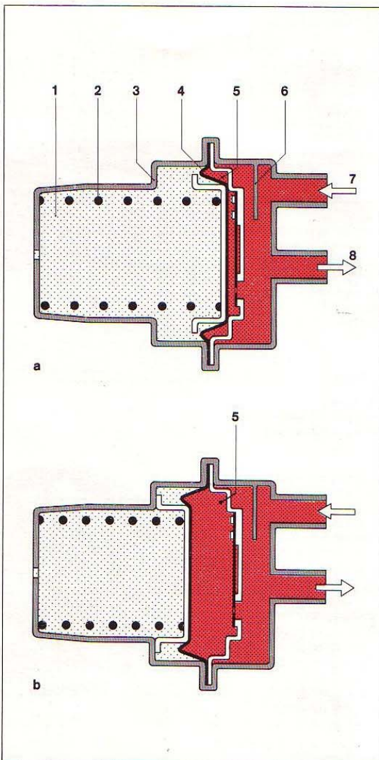
8. ábra. Nyomástároló a) üresen b) feltöltve
