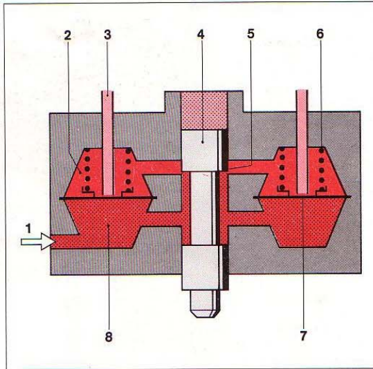
20. ábra. Üzemanyag-elosztó a nyomásszabályozó szelepekkel
