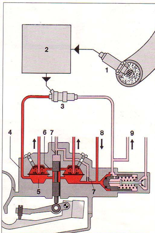
37. ábra. Kiegészítő alkatrészek a lambda-szabályozáshoz
