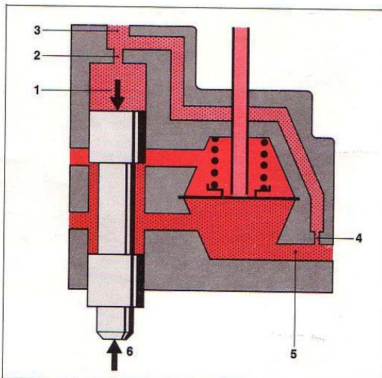
18. ábra. Rendszernyomás és vezérlőnyomás
