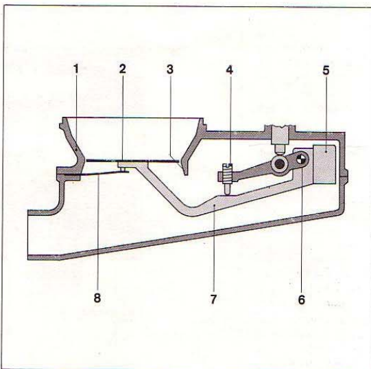
12. ábra. Légmennyiségmérő nyugalmi helyzetben
