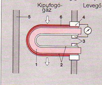
41. ábra. A lambda-szonda elhelyezése a kipufogócsőben (vázlatosan)
