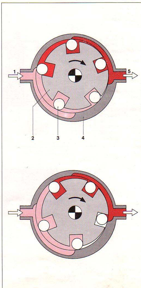
7. ábra. Görgőcellás szivattyú. Működési elv 1 Szívóoldal 2 Forgótárcsa 3 Görgő 4 Szivattyúház 5 Nyomóoldal Nyomásmentes üzemanyag Üzemanyag-szállítás iránya Üzemanyag nyomás alatt
