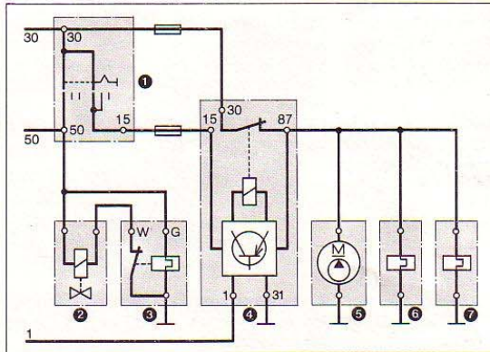
39. ábra. Motorindítás (hideg motor) Hidegindító szelep és a hő - idő kapcsoló bekapcsolva. A motor forogni kezd (impulzusok a gyújtótekercs 1 kapcsán). Üzemanyag-szivattyú, pótlevégőretesz és a melegésszabályozó működik
