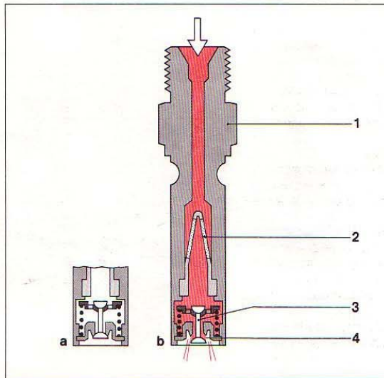
11. ábra. Befecskendező szelep
