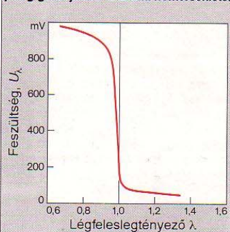
40. ábra. A lambda-szonda feszültség-jelleg-görbéje 600°C üzemi hőmérsékleten
