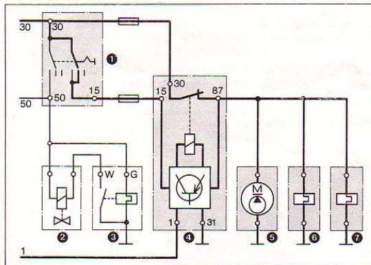
40. ábra. Üzem Gyújtás bekapcsolva, a motor jár. Vezérlőrelé, üzemanyag-szivattyú, pótlevégőretesz és a melegésszabályozó bekapcsolva
