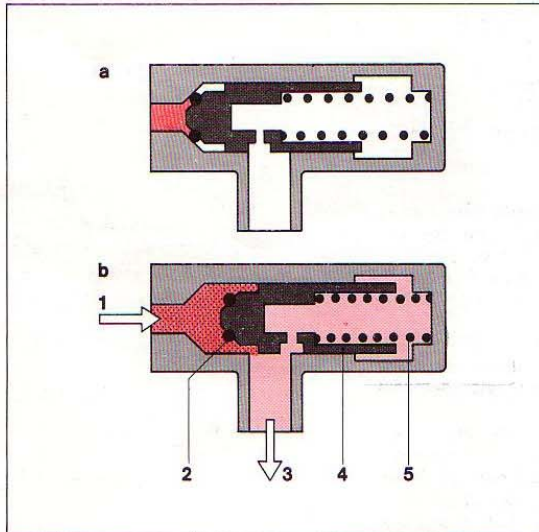
10. ábra. Nyomásszabályozó az üzemanyag-elosztón
