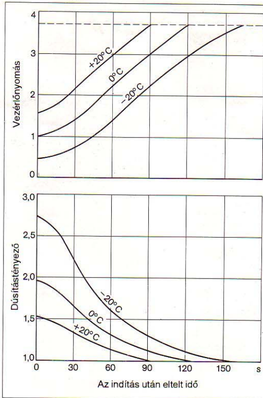
27. ábra. A melegedésszabályozó jelleggörbéi különböző motorhőmérsékleten. Az 1,0 dúsítástényező megfelel az üzemi üzemanyag-adagolásának.
