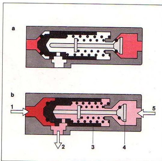
19. ábra. Nyomásszabályozó az ütközőszeleppel a) nyugalmi helyzetben b) üzemi helyzetben
