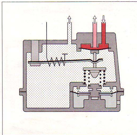
35. ábra. Melegedésszabályozó (vezérlőnyomás-szabályozó) a teljes terhelés-membránnal, teljes terhelésnél
