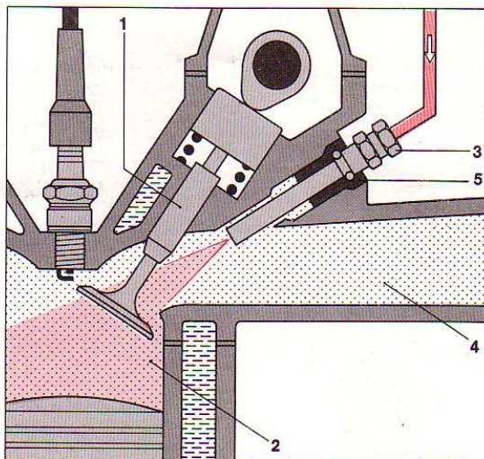
23. ábra. Keverékképzés 1 Szívószelep 2 Egéstér 3 Befecskendező szelep 4 Szívócső 5 Hőszigetelő rögzítőhüvely
