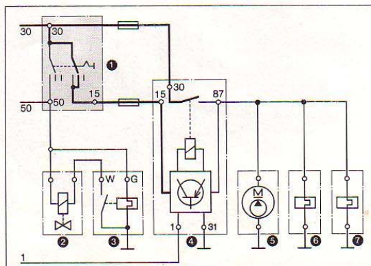
41. ábra. Gyújtás bekapcsolva, a motor nem jár Nincs impulzus a gyújtótekercs 1 kapcsán. Vezérlőrelé, üzemanyag-szivattyú, pótlevégőretesz és a melegésszabályozó kikapcsolva
