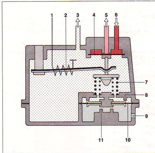
34. ábra. Melegedésszabályozó (vezérlőnyomás-szabályozó) a teljes terhelés-membránnal, alapjáratban és részterhelésnél
