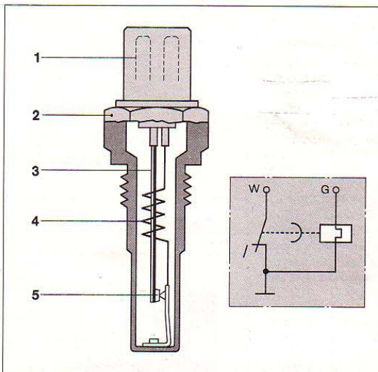
26. ábra. Hő-idő kapcsoló
