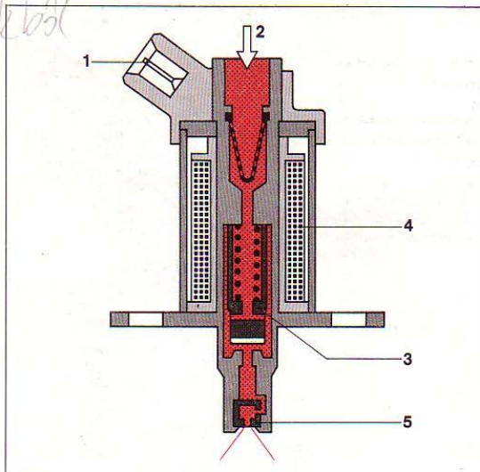
25. ábra. Hidegindító szelep működés közben
