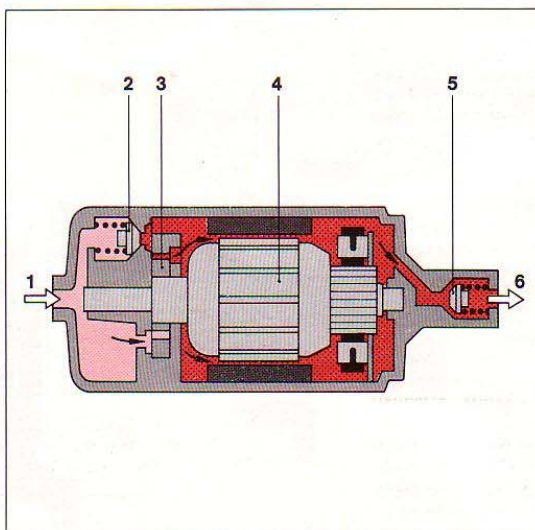
6. ábra. Üzemanyag-szivattyú 1 Szívóoldal 2 Nyomáshatároló szelep 3 Görgőcellás szivattyú 4 Motor forgórésze 5 Visszacsapószelep 6 Nyomóoldal
