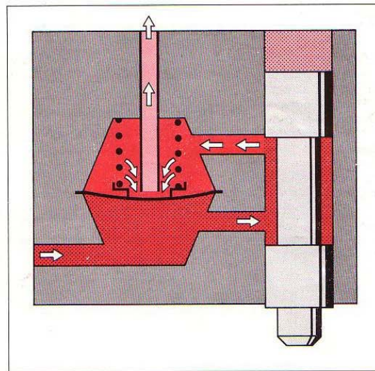
21. ábra. A nyomásszabályozó szelep állása sok üzemanyag befecskendezése esetén
