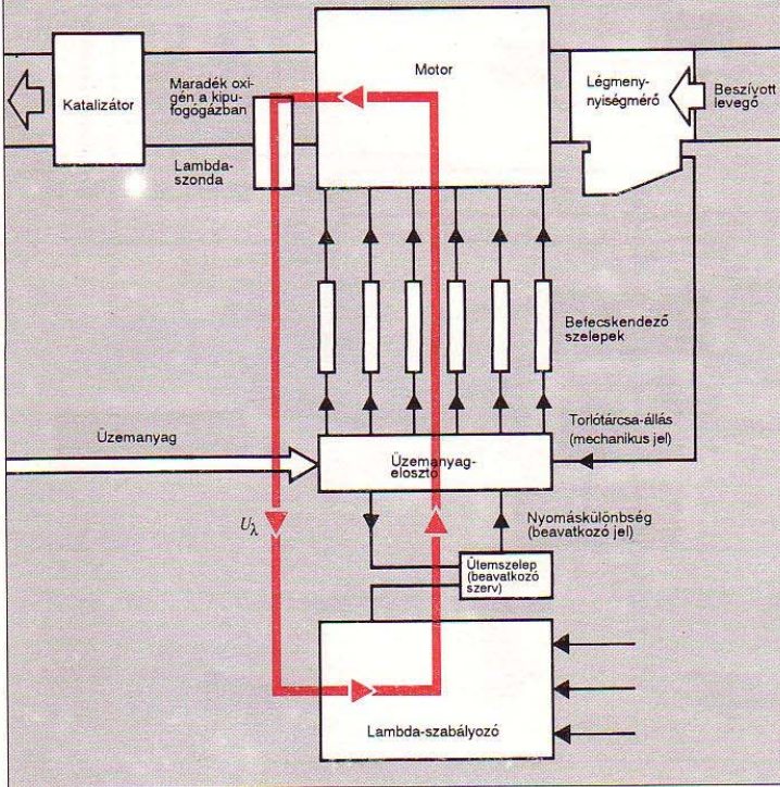
44. ábra. Lambda-szabályozókör
