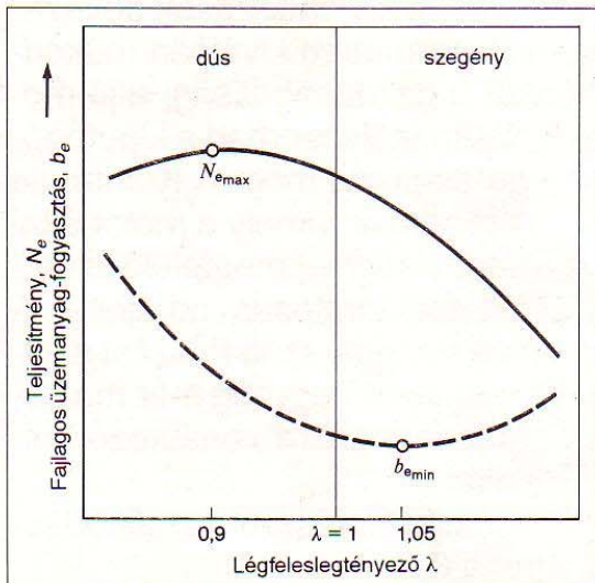
2. ábra. A légfeslegtényező befolyása a teljesítményre és a fajlagos üzemanyag-fogyasztásra
