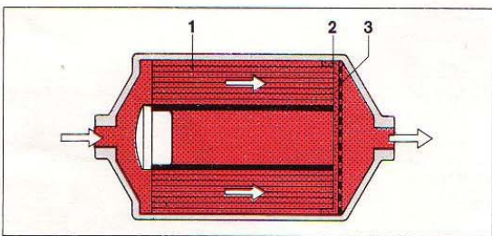
9. ábra. Üzemanyagszűrő 1 Papírszűrő 2 Szita 3 Támasztólap
