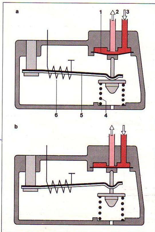
28. ábra. Melegedésszabályozó
