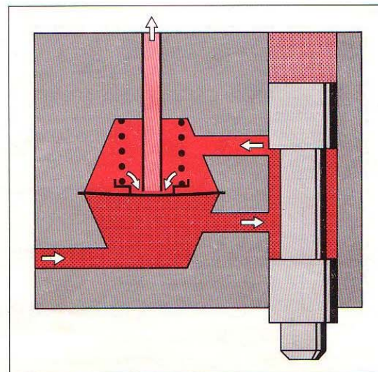
22. ábra. A nyomásszabályozó szelep állása kevés üzemanyag befecskendezése esetén
