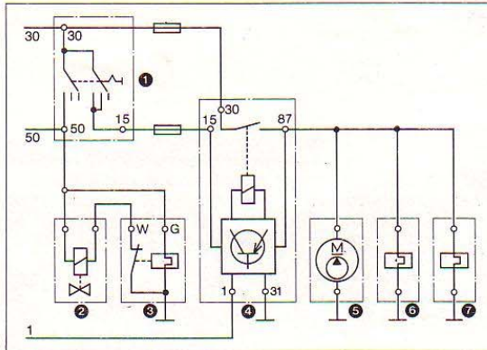
38. ábra. Kapcsolás nyugalmi helyzetben 1 Gyújtáskapcsoló 2 Hidegindító szelep 3 Hő - idő kapcsoló 4 Vezérlőrelé 5 Üzemanyag-szivattyú 6 Melegésszabályozó 7 Pótlevégőretesz
